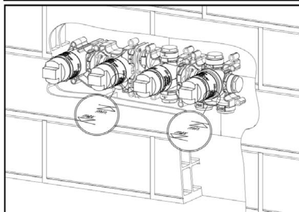
(B) Montage im Mauerwerk Solid wall mounting
